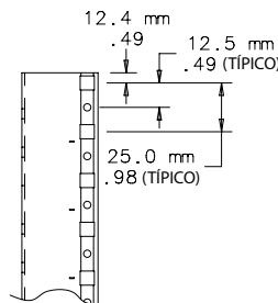
DETALLE
