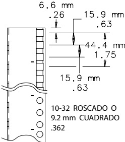
DETALLE
